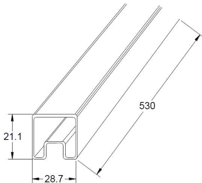
Tube: 530*28.7*21.1mm
